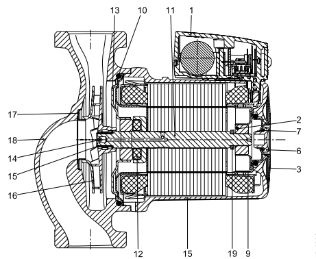
Рис. 34. Насос UPS, модели UPS xx-100
