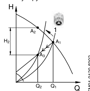
Регулируемый насос
