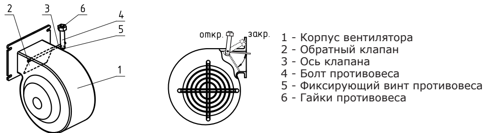
Рис.6 Вентилятор наддува
